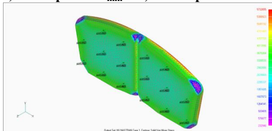
Gambar 21. Hasil simulasi Tegangan Thermal sepatu rem model 2 dengan ketebalan 5mm dilihat dari samping
