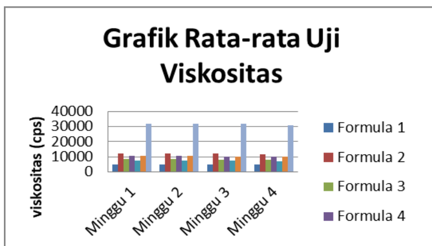
Gambar.3 Hasil viskositas
