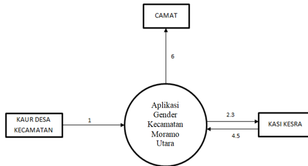
Gambar 3. Diagram Konteks
