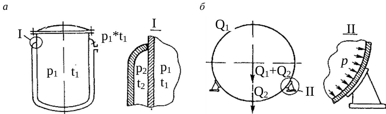
Рисунок 8.3 – Приклади зміни навантажень, що діють на оболонки: а – з'єднання корпусу апарата з оболонкою; б – з'єднання оболонки з опорними пристроями
