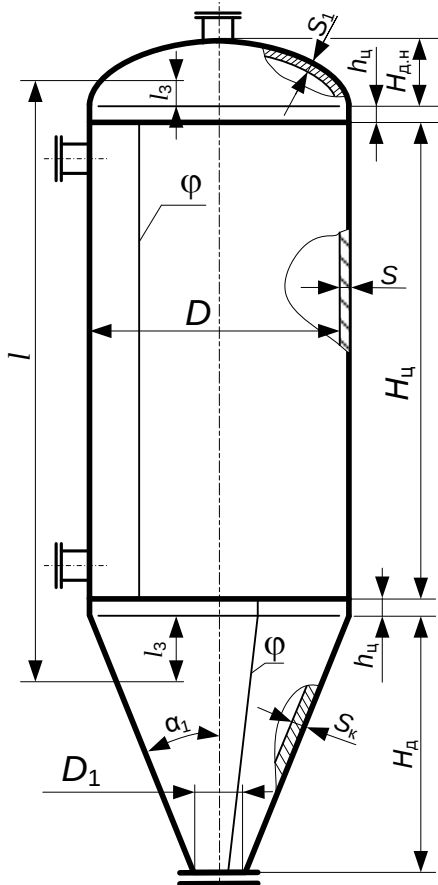
Рисунок 10.4 – Корпус апарата
