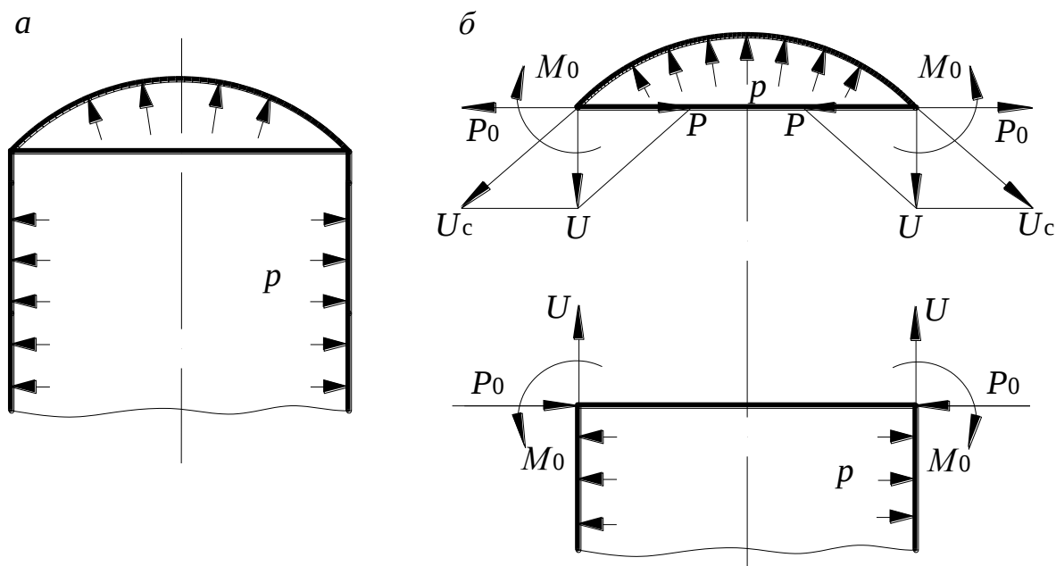
Рисунок 8.5 – Схема для визначення крайових сил і моментів:
