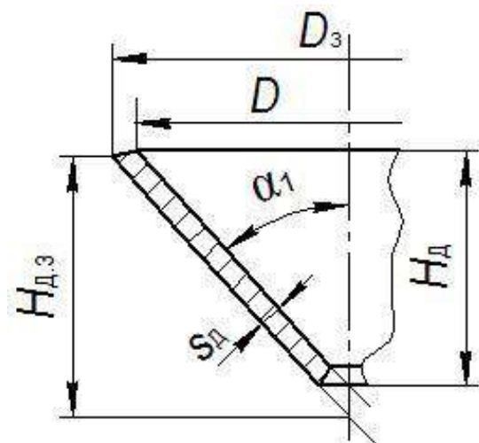
Рисунок 9.1 – Конструкції днищ зварних сталевих апаратів:
