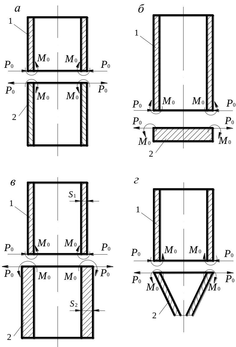
Рисунок 8.4 – Крайові сили і моменти (продовження): в, г – зміна геометричних розмірів (форми) оболонки при переході від одного перерізу до іншого
