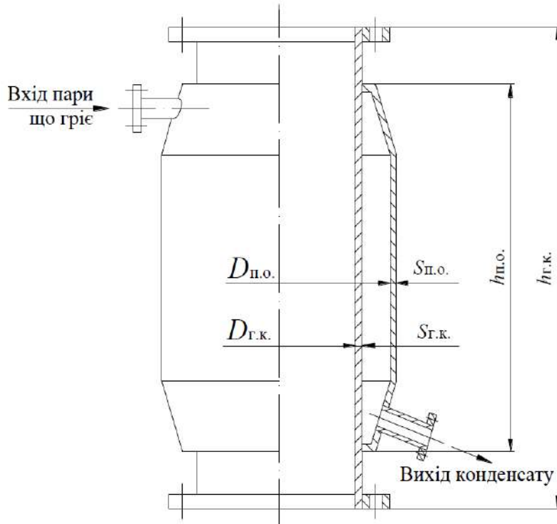
Рисунок 10.1 – Вертикальний роторно-плівковий апарат з паровим обігрівом
