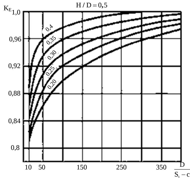
Рисунок 9.6 – Графік для визначення коефіцієнта K_E
