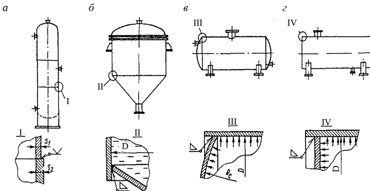
Рисунок 8.2 – Приклади зміни геометричних розмірів оболонок:
