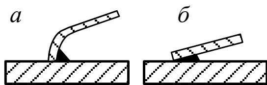
Рисунок 1.5 – Доступність шва для зварювання:
