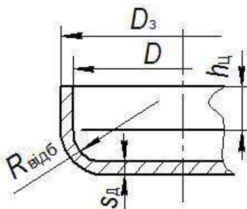
Рисунок 9.1 – Конструкції днищ зварних сталевих апаратів:
