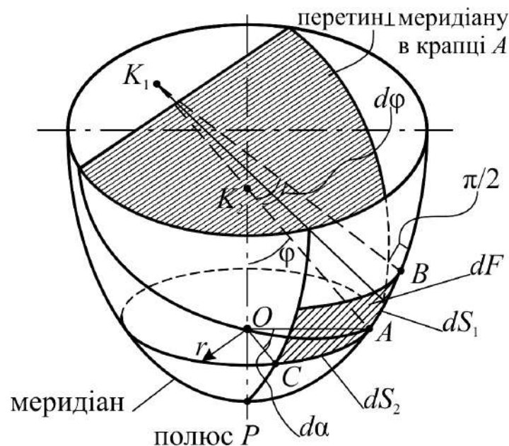
Рисунок 2.3 – Оболонка обертання
