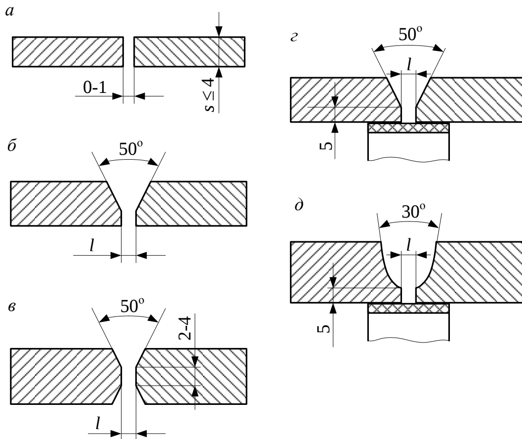
Рисунок 1.2 – Підготовка кромки для автоматичного зварювання під шаром флюсу: а – безскісна підготовка кромки; б – одностороння обробка кромки; в – двостороння обробка кромки; г і д – зварка на підкладному кільці
