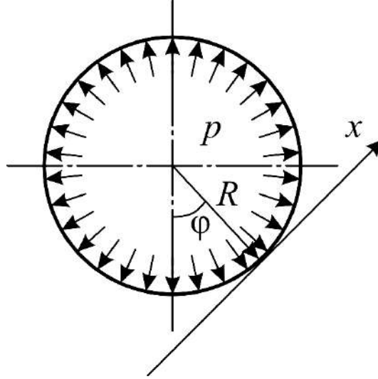
Рисунок 3.19 – Сферичний елемент, навантажений внутрішнім газовим тиском p
