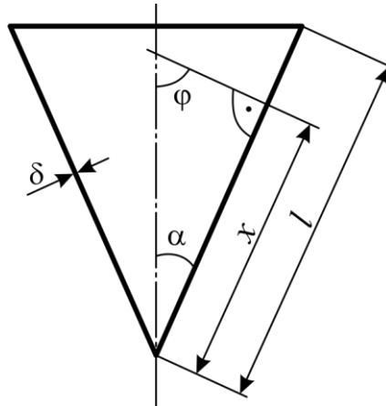
Рисунок 3.20 – Конічна оболонка
