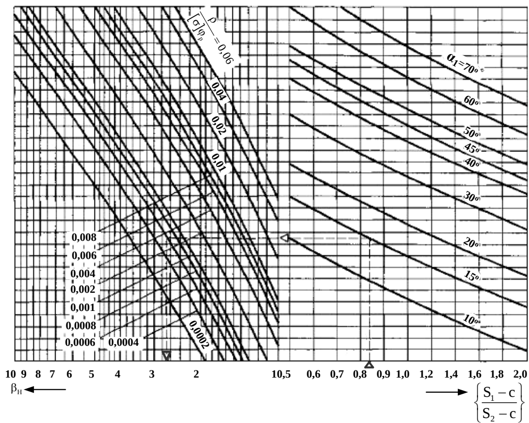
Рисунок 9.27 – Діаграма для визначення коефіцієнта \beta_H при розрахунку товщини стінок переходів обичайок
