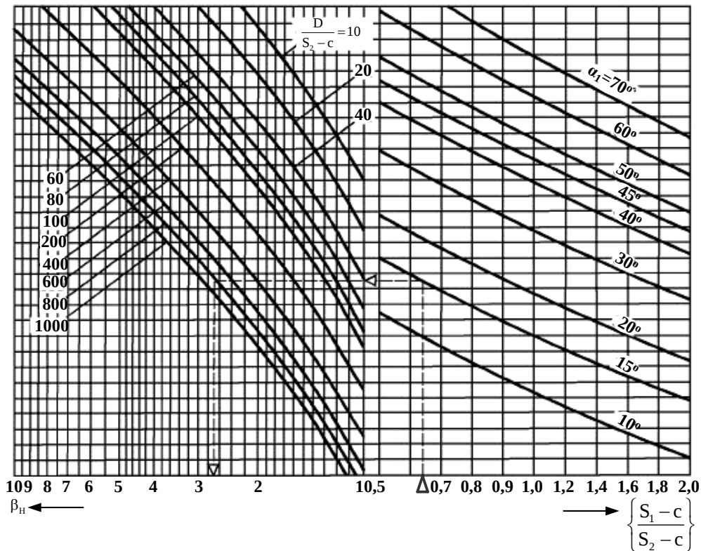
Рисунок 9.28 – Діаграма для визначення коефіцієнта \beta_H при виконанні перевірного розрахунку
