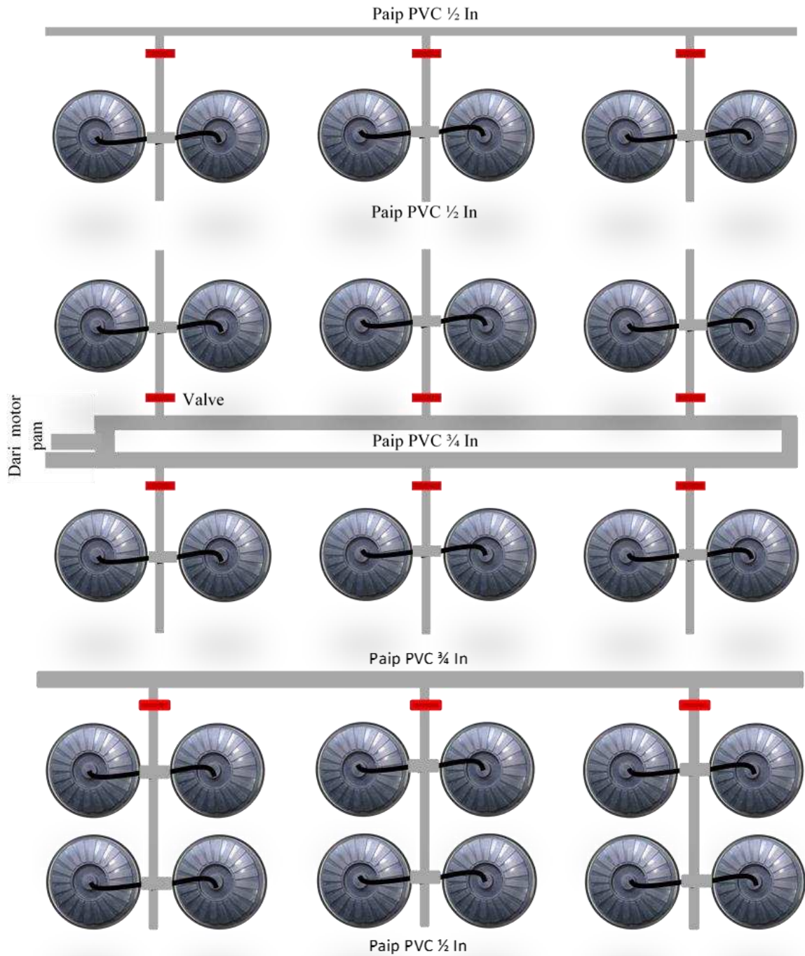
Rajah 6. Cadangan susunan bekas-bekas tong dalam mesin Auto-PT
