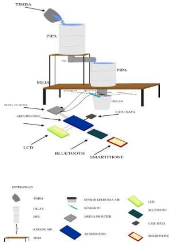
Gambar 1. perancangan Alat
