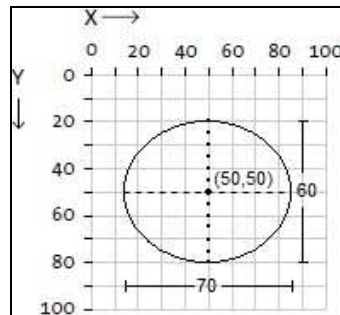
Gambar 15. Sistem Koordinat Ellips dengan Titik Koordinat (50, 50), Lebar 70 Piksel, dan Tinggi 60 Piksel
