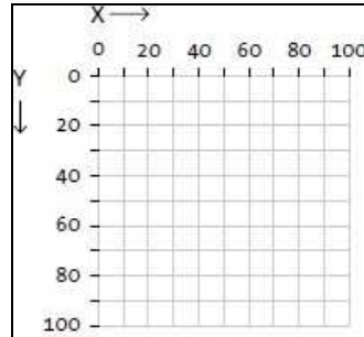
Gambar 3. Sistem Koordinat pada Display Window dengan Lebar 100 Piksel dan Tinggi 100 Piksel [5]
