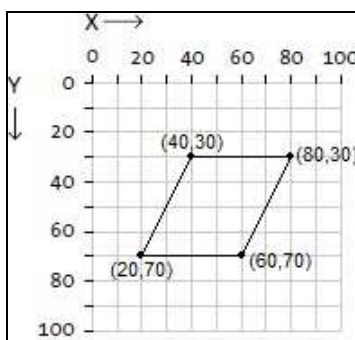
Gambar 11. Sistem Koordinat Jajaran Genjang dengan Titik-Titik Koordinat: (40, 30), (80, 30), (60, 70), dan (20, 70)
