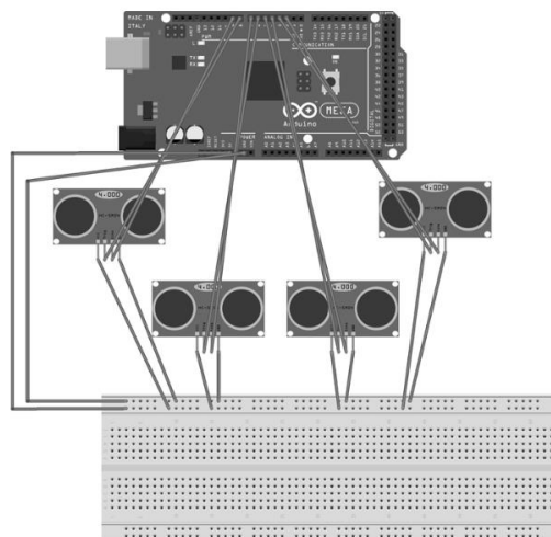
Gambar 4. Rangkaian Arduino dengan sensor HC-SR04
