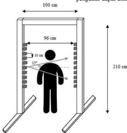
Gambar 1. Rancangan Alat Pengukur
