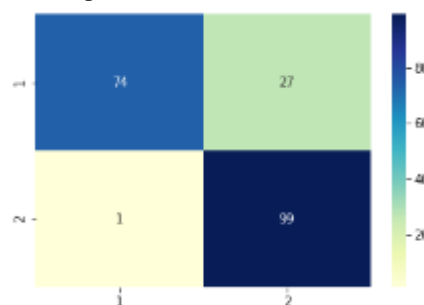
Gambar 16. Confusion Matrik SVM Semua Variabel
