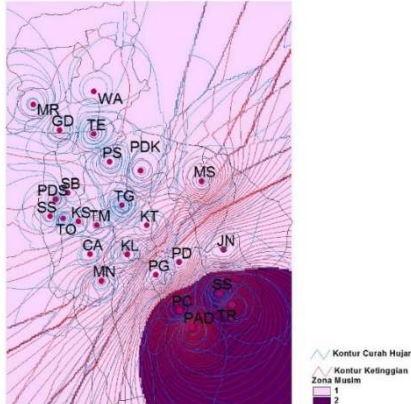
Gambar 15 Pengelompokan Zona Musim Menggunakan Jarak DTW dengan Faktor 1
