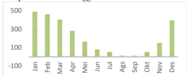
Gambar 18. Pola Curah Hujan Zona Musim 2 dengan Jarak DTW
