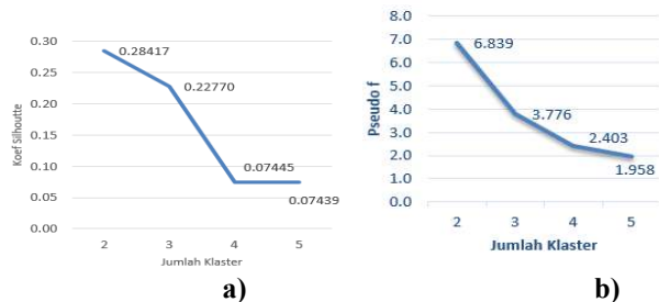
Gambar 14 (a) Koefisien Silhouette dan (b) Nilai Pseudo-f Statistics Hasil Pengelompokan dengan Jarak DTW
