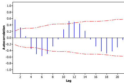
Gambar 7 ACF Data Curah Hujan Sukosari
