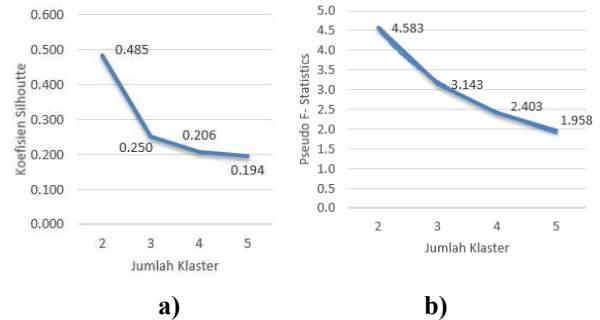
Gambar 8 (a) Koefisien Silhouette dan (b) Nilai Pseudo-f Statistics Hasil Pengelompokan dengan Jarak ACF
