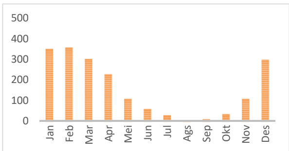
Gambar 11 Pola Curah Hujan Zona Musim 1 dengan Jarak ACF
