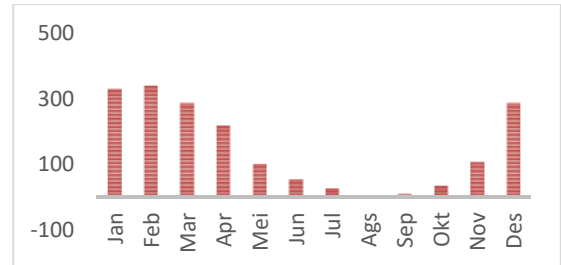
Gambar 17. Pola Curah Hujan Zona Musim 1 dengan Jarak DTW
