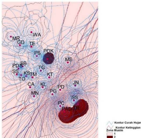
Gambar 10 Pengelompokan Zona Musim Menggunakan Jarak ACF Pada Faktor 3
