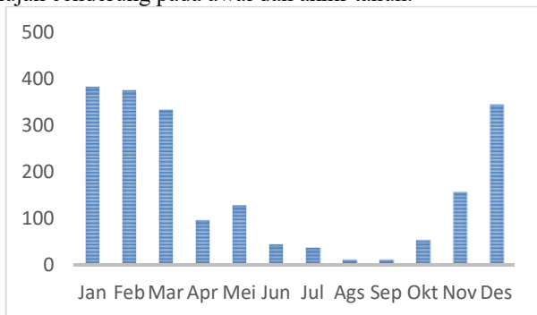
Gambar 12 Pola Curah Hujan Zona 2 Pada Klaster dengan Jarak ACF
