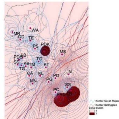
Gambar 9 Pengelompokan Zona Musim Menggunakan Jarak ACF Pada Faktor 1
