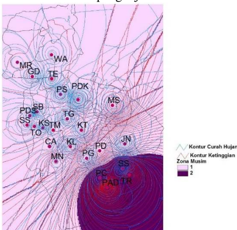
Gambar 16. Pengelompokan Zona Musim Menggunakan Jarak DTW dengan Faktor 3
