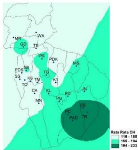
Gambar 2 Rata – rata Curah Hujan di Mojokerto
