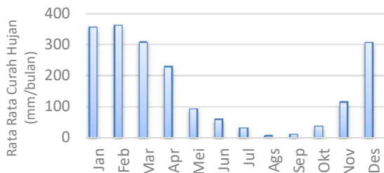
Gambar 3 Rata- rata Curah Hujan di Mojokerto
