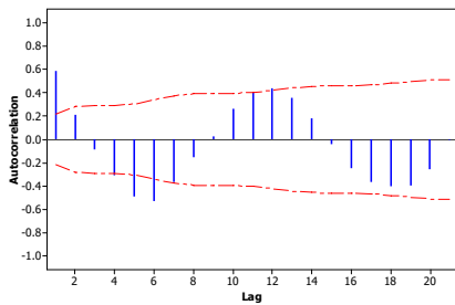
Gambar 6. ACF Data Curah Hujan Trowulan
