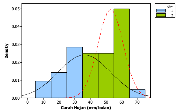
Gambar 19 Perbandingan Rata Rata Curah Hujan Zona 1 dan Zona 2 dengan Jarak DTW
