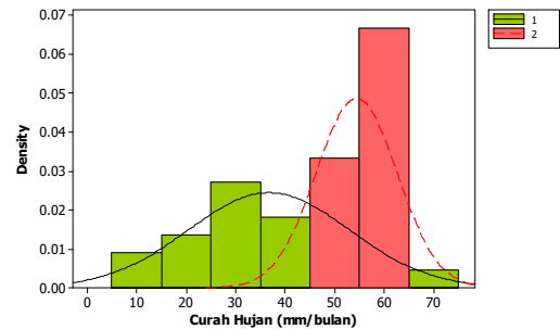
Gambar 13 Perbandingan Rata Rata Curah Hujan Zona 1 dan Zona 2 dengan Jarak ACF
