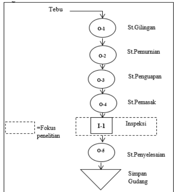
Gambar 2. 2 Diagram proses operasi produksi gula kristal putih
