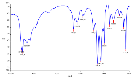
Gambar 4. Spektrum FTIR kolagen
