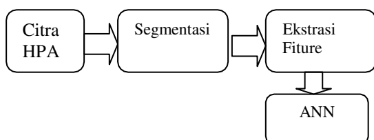
Gambar 3.1 Metodologi Penelitian
