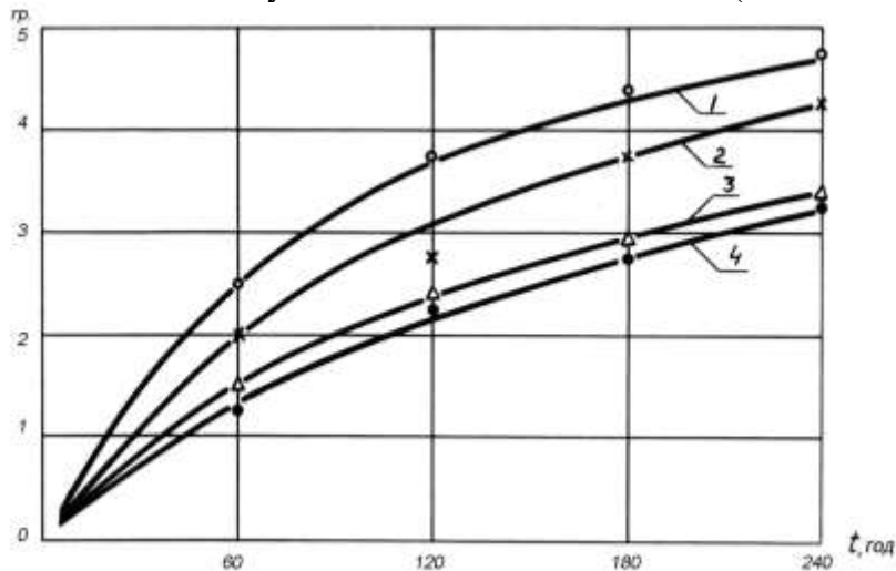
Рис. 2. Знос деталей двигунів тракторів при експлуатаційних випробуваннях: 1, 2 – серійними центрифугами, 3, 4 – пропонуєміми центрифугами
