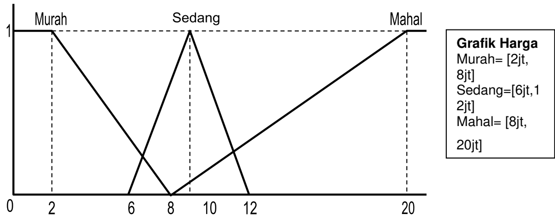
Gambar 1 Fungsi keanggotaan variabel harga mahal
