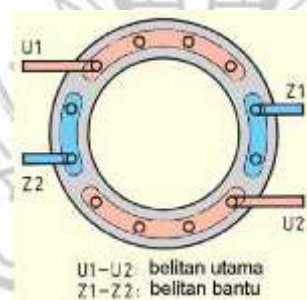
Gambar 1. Medan Magnet Utama dan Medan magnet Bantu pada Motor Satu Fasa http://siapbelajar.com/wp-content/uploads/2013/09/6_102Teknik-Listrik-Indus-Jilid-2.pdf
