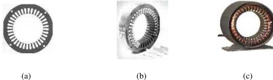
Gambar 3. Komponen Stator
