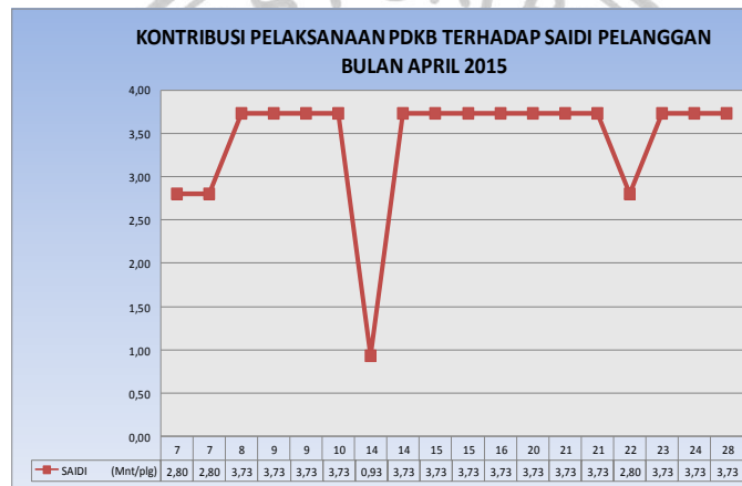
Gambar 2. Grafik Kontribusi Pelaksanaan PDKB terhadap SAIDI Pelanggan
