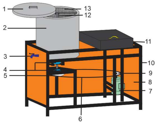
Gambar 3. Gambar konstruksi mesin peniris yang akan diwujudkan.
