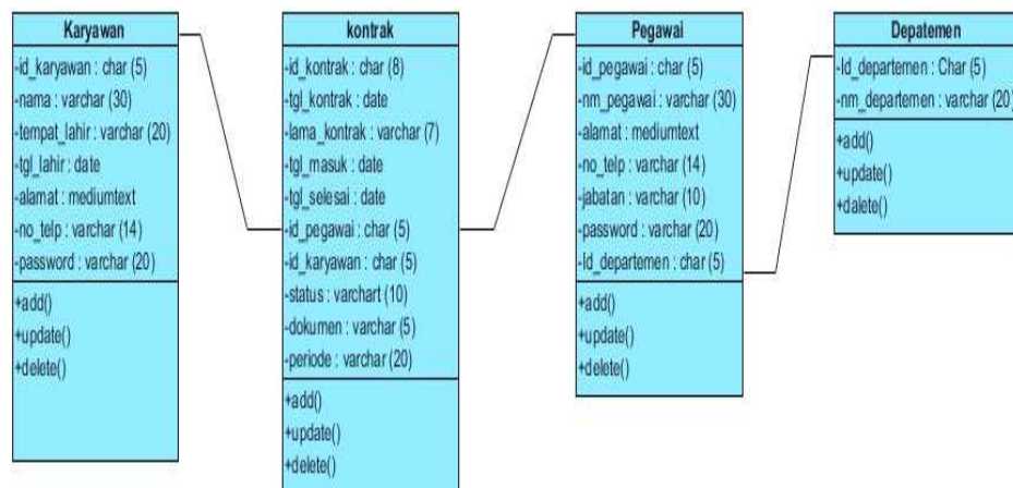
Gambar 4. Class Diagram Yang Diusulkan
