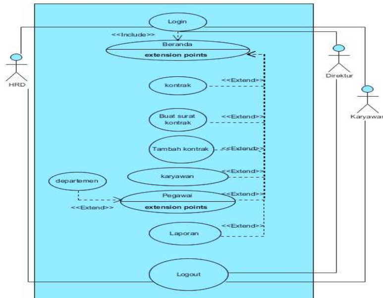
Gambar 1. Use Case Diagram Yang Diusulkan Untuk Sistem Kontrak
