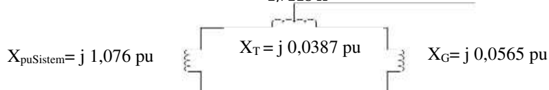
■ Gambar 11. Rangkaian ekivalen impedansi urutan positif untuk gangguan didalam zona proteksi pada sisi 16,5 kV
