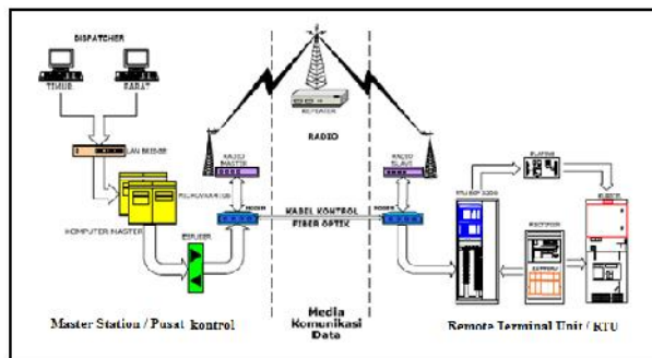
Arsitektur SCADA
