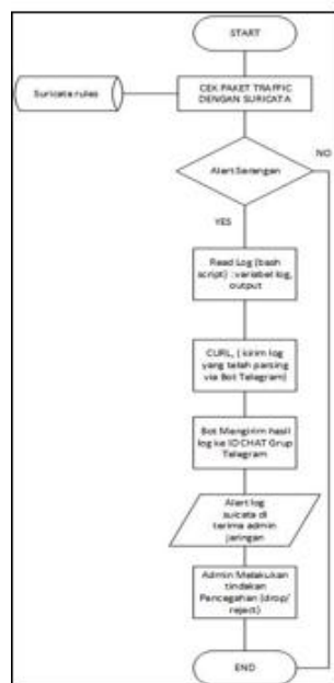
Gambar 2. Flowchat Cara Kerja Suricata (IDS) dan Bot
