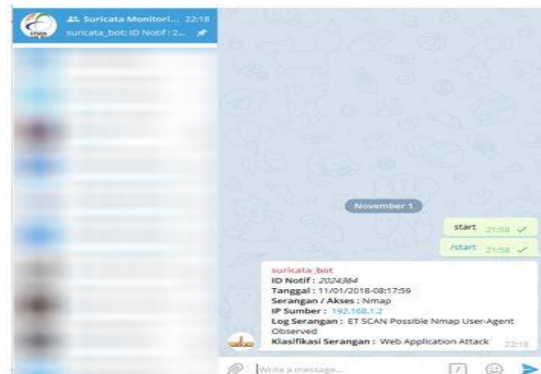
Gambar 5. Log Suricata Nmap ke Telegram
