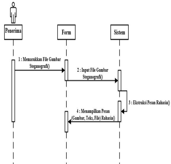
Gambar 10. Sequential Diagram Proses Ekstraksi Aplikasi Steganografi
