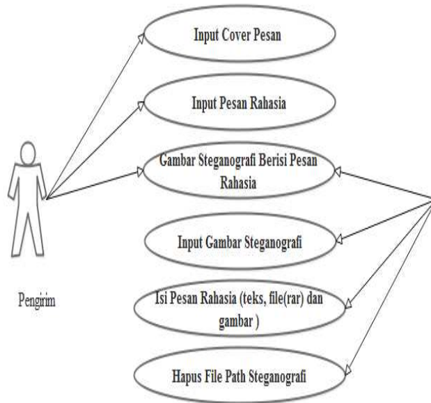
Gambar 6. Use Case Diagram Aplikasi Steganografi
