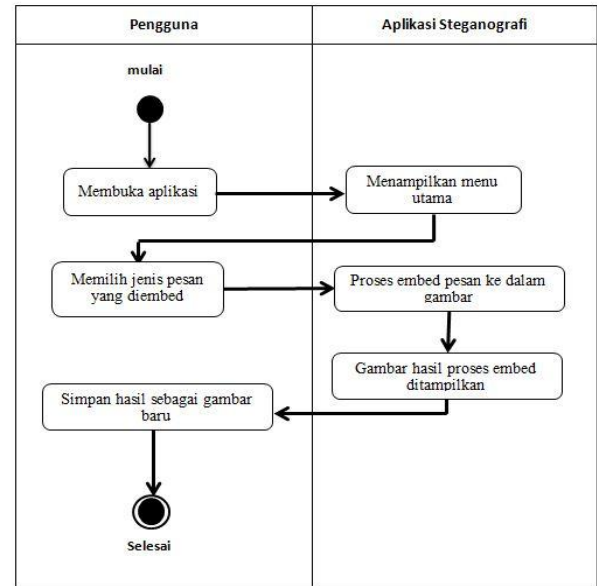
Gambar 7. Activity Diagram Proses Embed Aplikasi Steganografi
