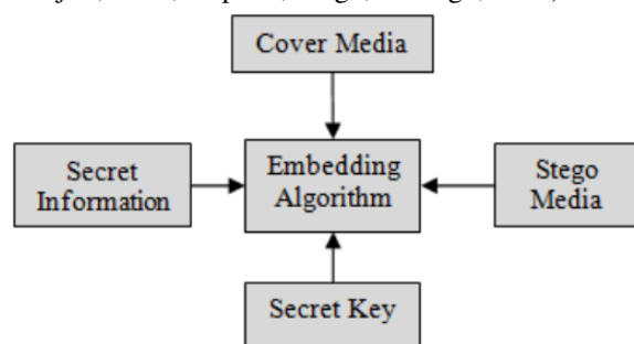
Gambar 1. Proses Steganografi
