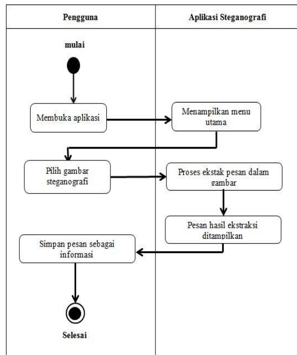
Gambar 8. Activity Diagram Proses Ekstrak Aplikasi Steganografi
