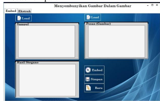
Gambar 13. Form Menyembunyikan Pesan Gambar di dalam Gambar
