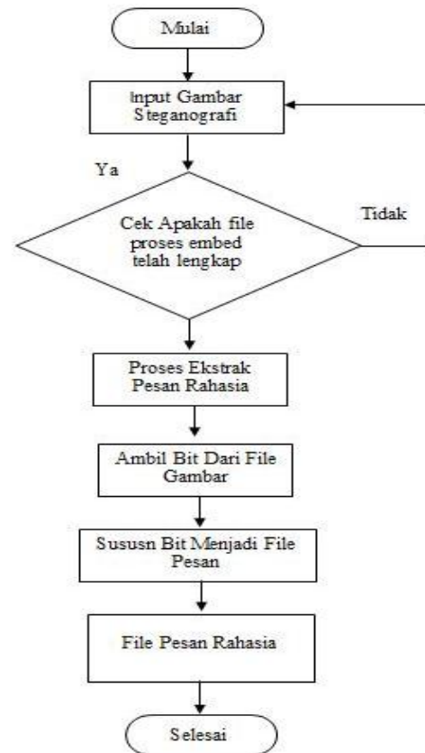
Gambar 5. Flowchart Ekstraksi Pesan Rahasia
