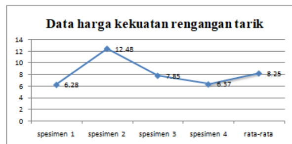
Gambar 4.6 Grafik Data harga kekuatan regangan tarik
