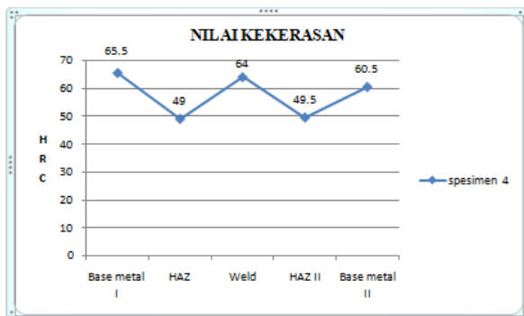
Gambar 4.4 Grafik nilai kekerasan spesimen 4
