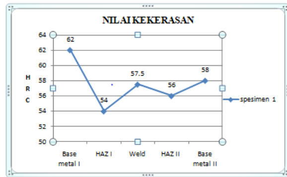
Gambar 4.1 Grafik nilai kekerasan specimen 1
