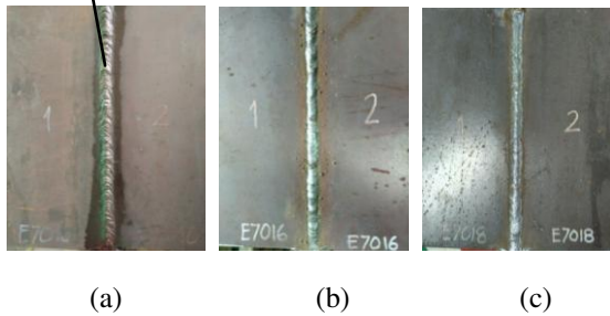
Gambar 6. Hasil pengelasan menggunakan: (a) elektroda E7010-P1, (b) elektroda E7016, (c) elektroda E7018
