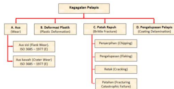
Gambar 2. Diagram Spektrum Kegagalan Pahat[4]
