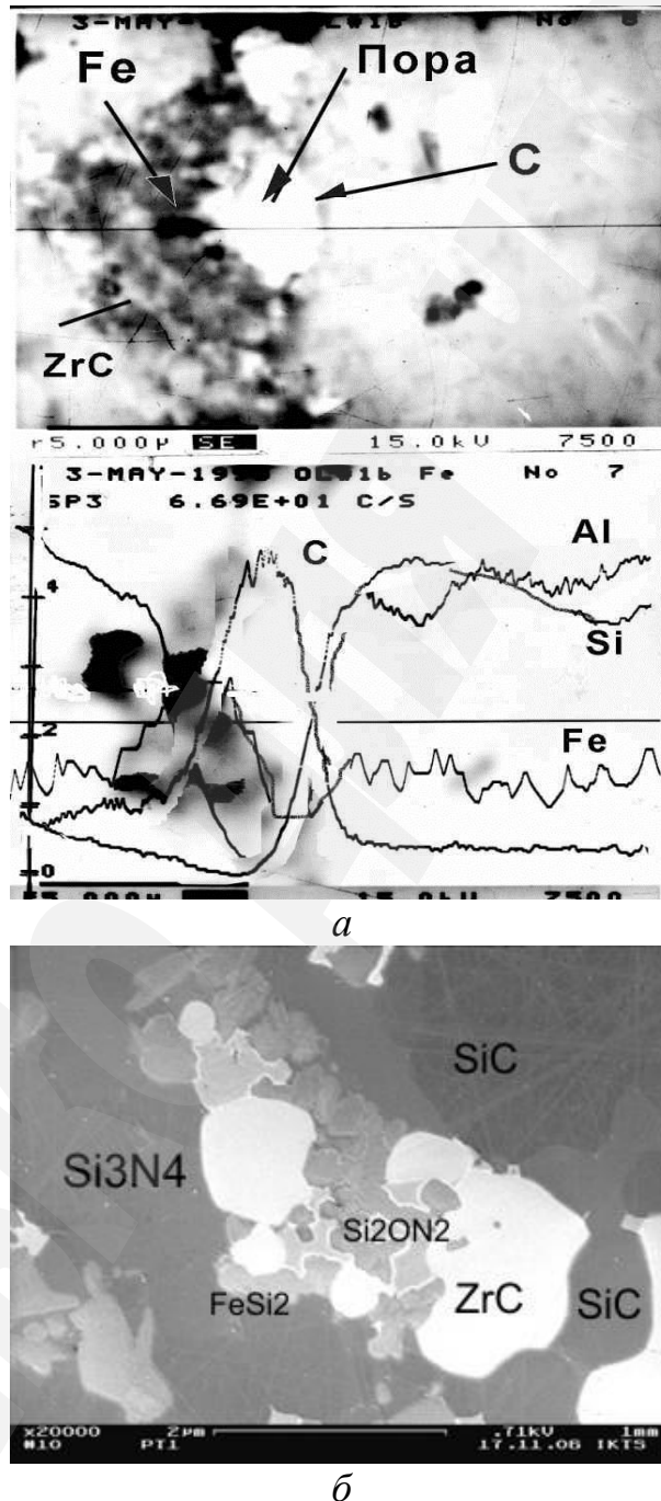
Рис. 2. Локалізація вуглецю на поверхні пори заготовки: а – за даними локального рентгеноспектрального аналізу; б – вигляд провідного кластеру термоелектричного композиту
