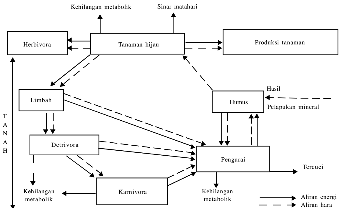
Gambar 1. Daur energi dan hara dalam ekosistem tanah (modifikasi dari Wallwork 1970).
