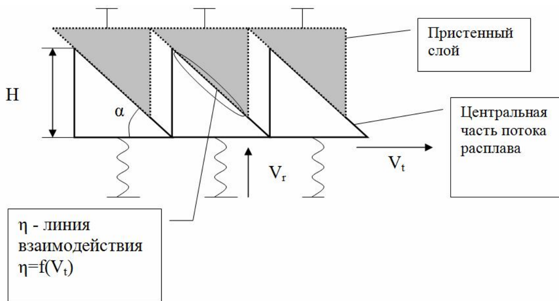
Рис. 3.14. Графическая интерпретация модели «пробкового» течения сжимаемой жидкости.
