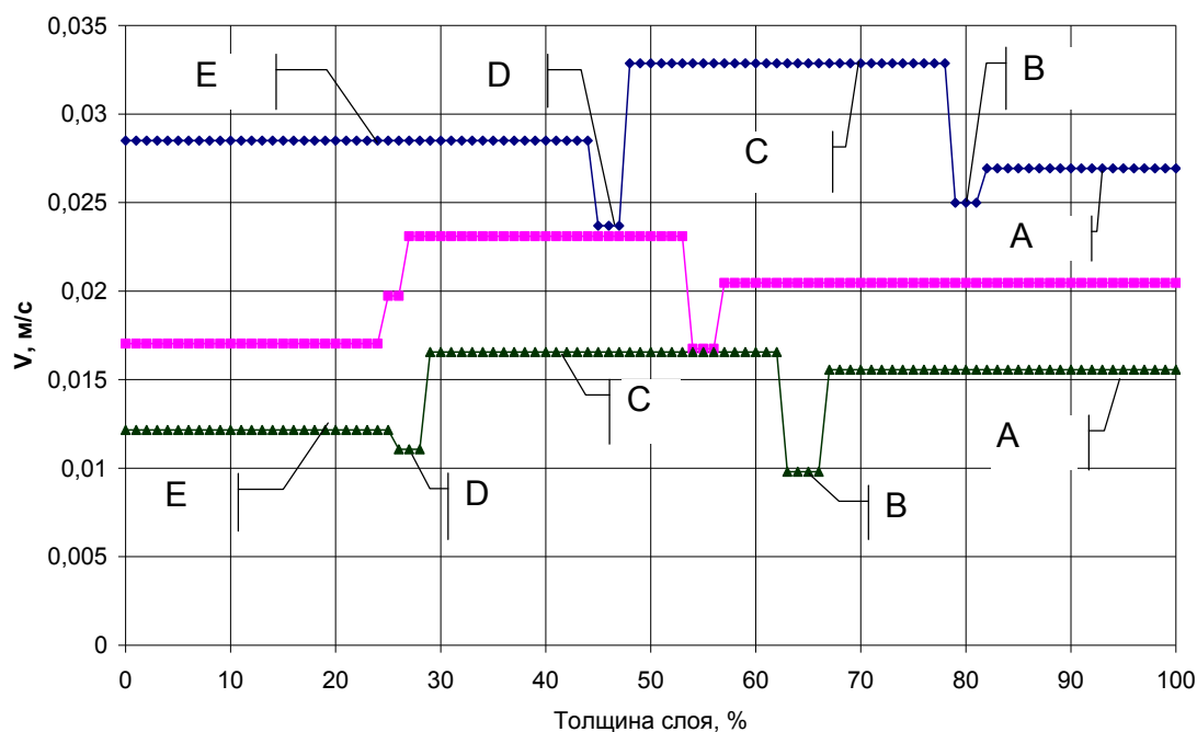
Рис. 4.3. Эпюра скоростей многослойных потоков построенная по экспериментальным результатам
