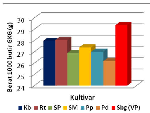
Gambar 5 dan 6. Grafik berat 1000 butir GKG dan produksi GKG/ha dari 6 kultivar padi sawah lokal Kaltim.
