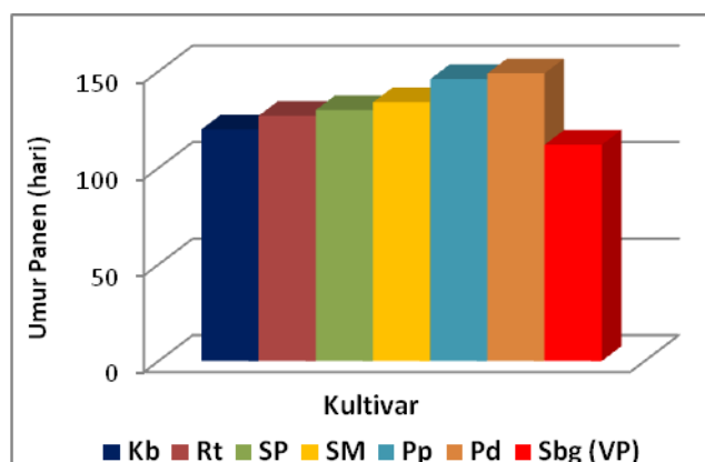
Gambar 7. Grafik umur panen dari 6 kultivar padi sawah lokal Kaltim
