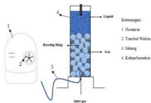
Gambar 1. Rangkaian alat ozonasi
