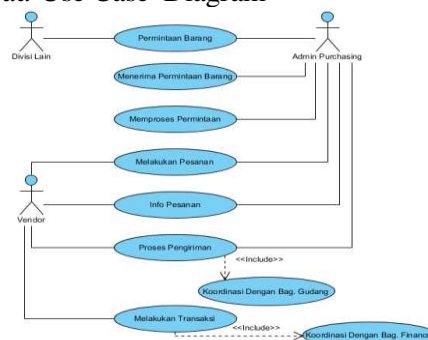
Gambar 1. Use Case Diagram Monitoring Permintaan Perlengkapan Peralatan Kantor
