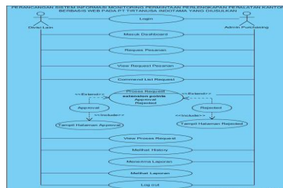
Gambar 4. Use Case Diagram Monitoring Permintaan Perlengkapan Peralatan Kantor
