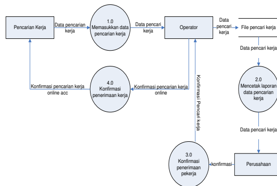
Gambar 3. DFD Sistem
