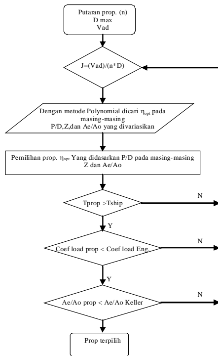
Gambar.2. Diagram alir pemilihan propeller
