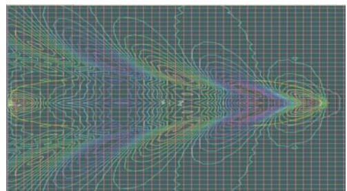
Gambar 11,- Perspektif Kontur Gelombang yang Terjadi (Tampak Atas)
