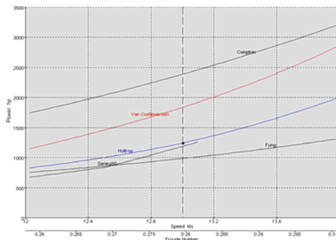
Gambar 2 Grafik Hubungan Speed (Froude Number) vs. Power Kapal BHO Pada Rentang Kecepatan 12-14 KNOTS
