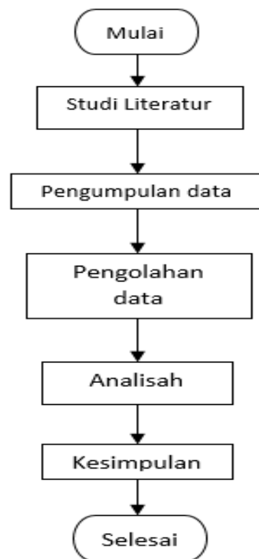
Gambar 3.1 Diagram alir
