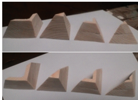
Gambar 4. Simulasi pemotongan dengan sudut yang berbeda dengan bidang setengah segi empat laminasi sebanyak dua lapis menggunakan lem PVaC (Sumber: Dokumentasi Tim Peneliti, 2018)
