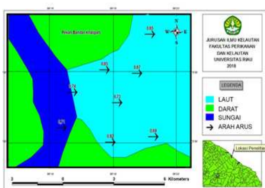
Gambar 2. Kecepatan Arus Saat Pasang Menuju Surut
