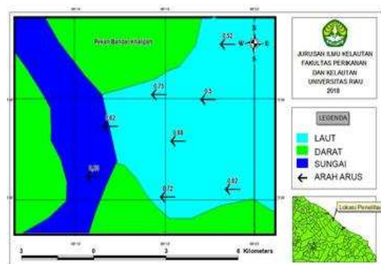
Gambar 3. Kecepatan Arus Saat Surut Menuju Pasang
