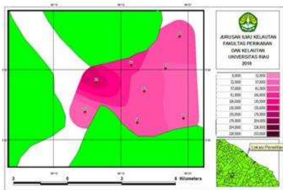
Gambar 6. Peta Sebaran Sedimen Tersuspensi bagian Middle Lier saat Pasang Menuju Surut.
