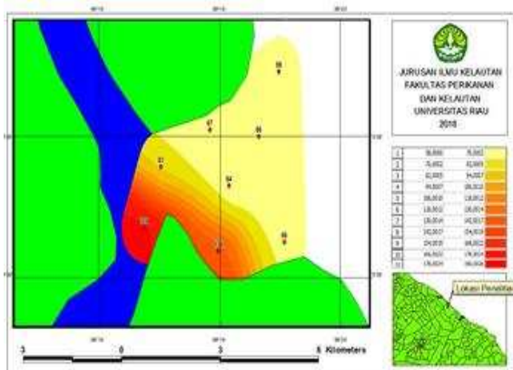
Gambar 10. Peta Rata rata Sebaran Konsentrasi Sedimen Tersuspensi (SSC) Pasang Menuju Surut
