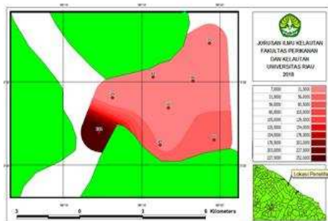
Gambar 4. Peta Sebaran Sedimen Tersuspensi bagian Upper Lier saat Pasang Menuju Surut
