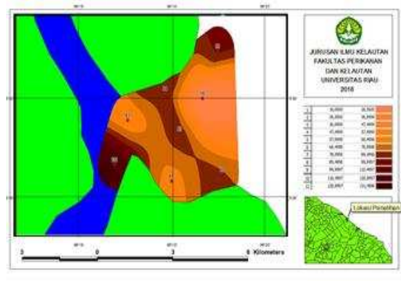
Gambar 11. Peta Rata rata Sebaran Konsentrasi Sedimen Tersuspensi (SSC) Surut Menuju Pasang.
