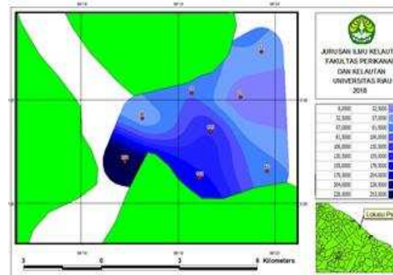
Gambar 9. Peta Sebaran Sedimen Tersuspensi bagian Lower Lier saat Surut Menuju pasang
