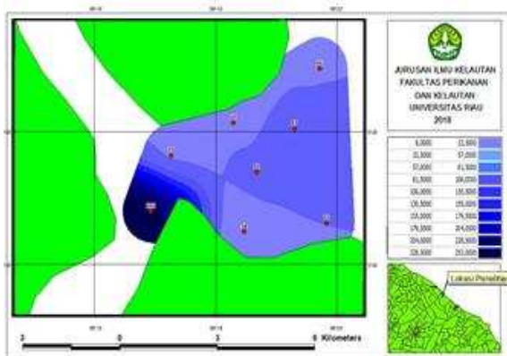
Gambar 8. Peta Sebaran Sedimen Tersuspensi bagian Lower Lier saat Pasang Menuju Surut.
