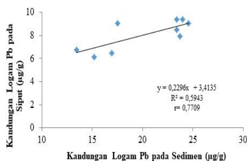
Gambar 4. Grafik Hubungan Kandungan Logam Pb pada Siput Sedut dengan Sedimen
