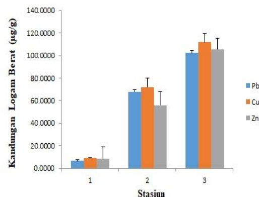
Gambar 2. Histrogram rata-rata kandungan logam Pb, Cu dan Zn pada siput Sedut
