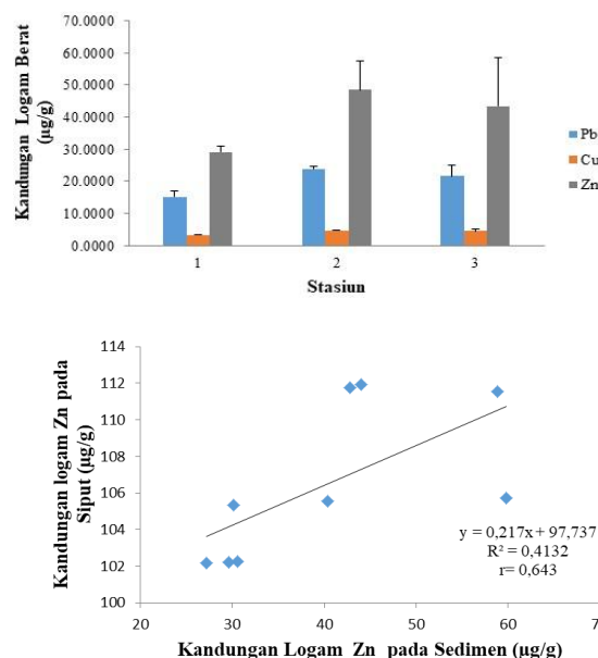
Gambar 3. Histogram Rata-rata konsentrasi logam Pb, Cu dan Zn pada Sedimen
