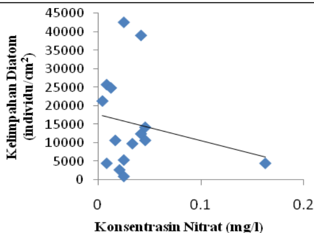
Gambar 3. Grafik Hubungan Kelimpahan Diatom dengan Konsentrasi Nitrat
