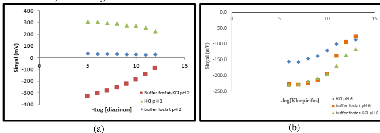
Gambar 1. Kurva hubungan antara -\log [diazinon] (a) dan -\log [klorpirifos] (b) terhadap sinyal
