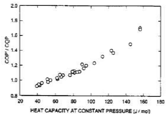
Gambar 3. Grafik Hubungan antara Kapasitas panas jenis Refrigeran terhadap Perubahan COP.
