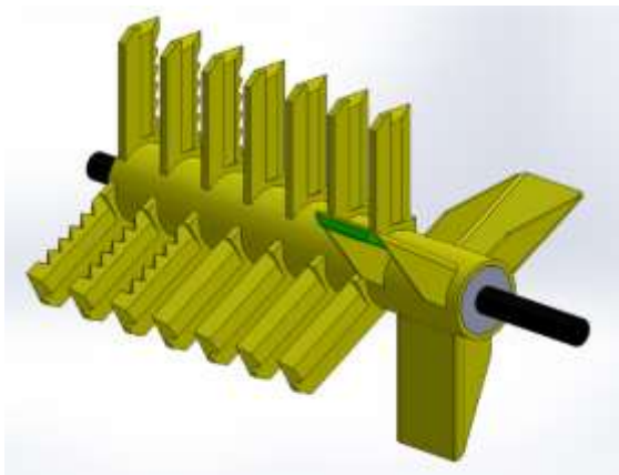
Gambar 7. Desain 3 dimensi bagian pencacahan
