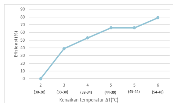
Gambar 2 Grafik efisiensi pada temperatur setting 50 °C terhadap kenaikan temperatur ( \Delta T )
