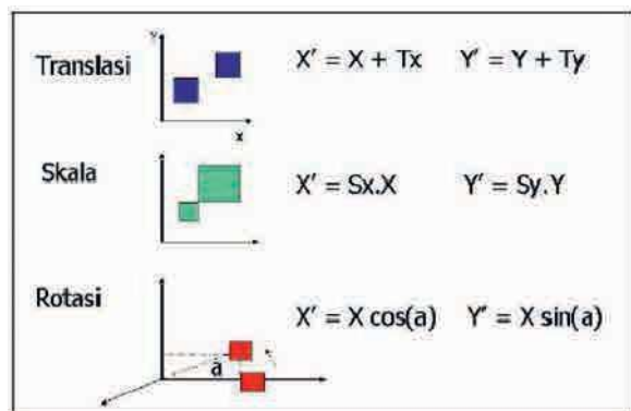
Gambar 4. Transformasi geometrik
