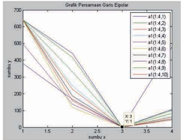
Gambar 11. Persamaan Garis Epipolar Kamera 5
