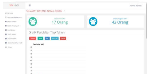
Gambar 1.8 Tampilan Beranda
