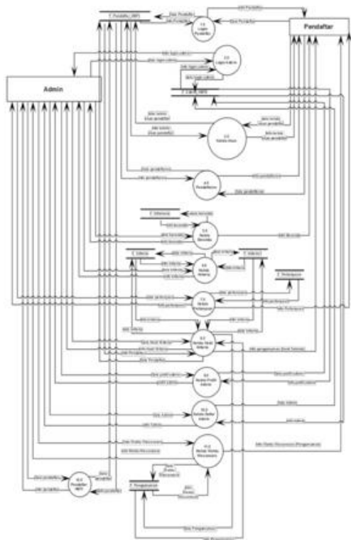
Gambar 1.5 DFD
