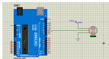
Gambar 15. Rangkaian Motor Servo
