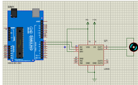
Gambar 16. Rangkaian Motor DC
