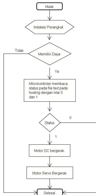
Gambar 4. Flowchart alat pengontrol pakan ikan lele
