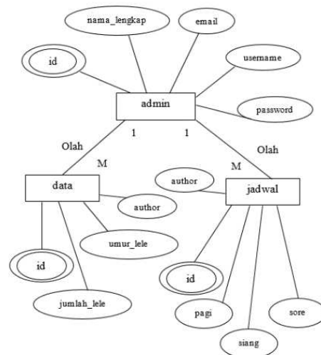
Gambar 19. ERD
