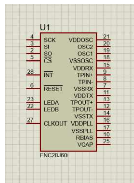
Gambar 14. Rangkaian Internet Shield
