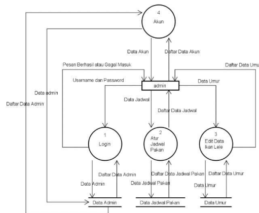
Gambar 18. DFD Level 1
