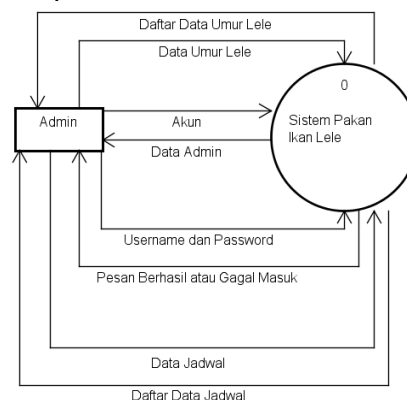
Gambar 17. DFD Level 0
