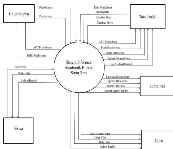
Gambar 2. Diagram konteks sistem yang diusulkan
