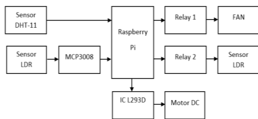
Gbr 5. Blok Diagram
