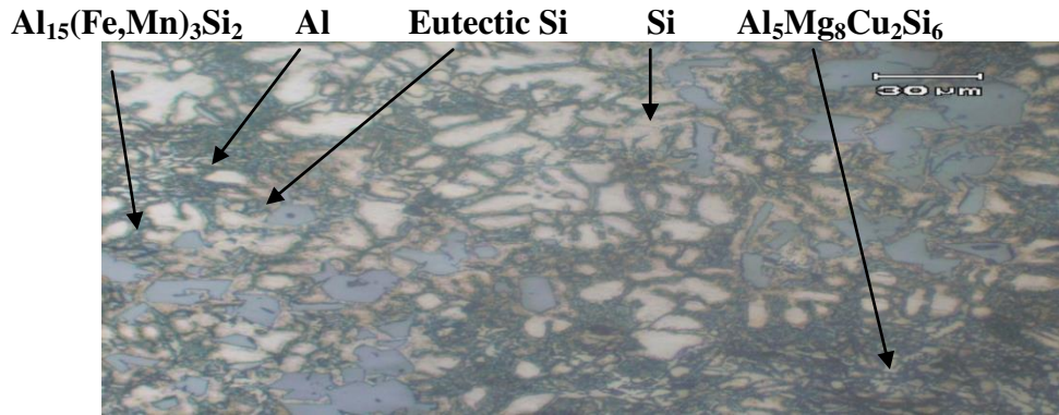
Gambar 5. Foto Struktur Mikro Blok Silinder Al-Si Tegak Lurus Dinding Liner dengan Etsa Kellers Reagent Pembesaran 400x.
